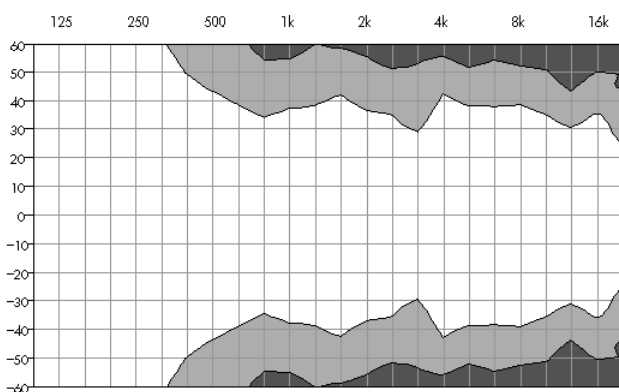
horizontal Isobarendiagramme C7-TOP
