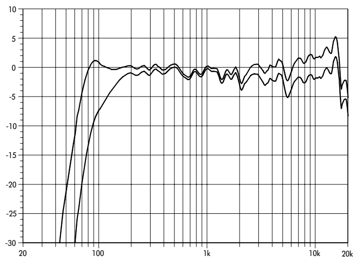
C7-TOP Frequenzgang, Standard, CUT- und HFA-Schaltung
