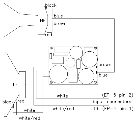
C7-TOP Verdrahtungsschema
